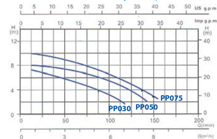
Curvas de rendimiento hidráulico Hydraulic performance curves
