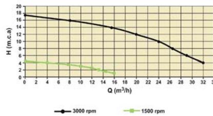
Curvas de rendimiento hidráulico Hydraulic performance curves
